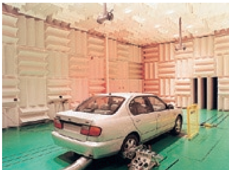
Innenansicht eines großen Reflexarmen Schallmessraumes
