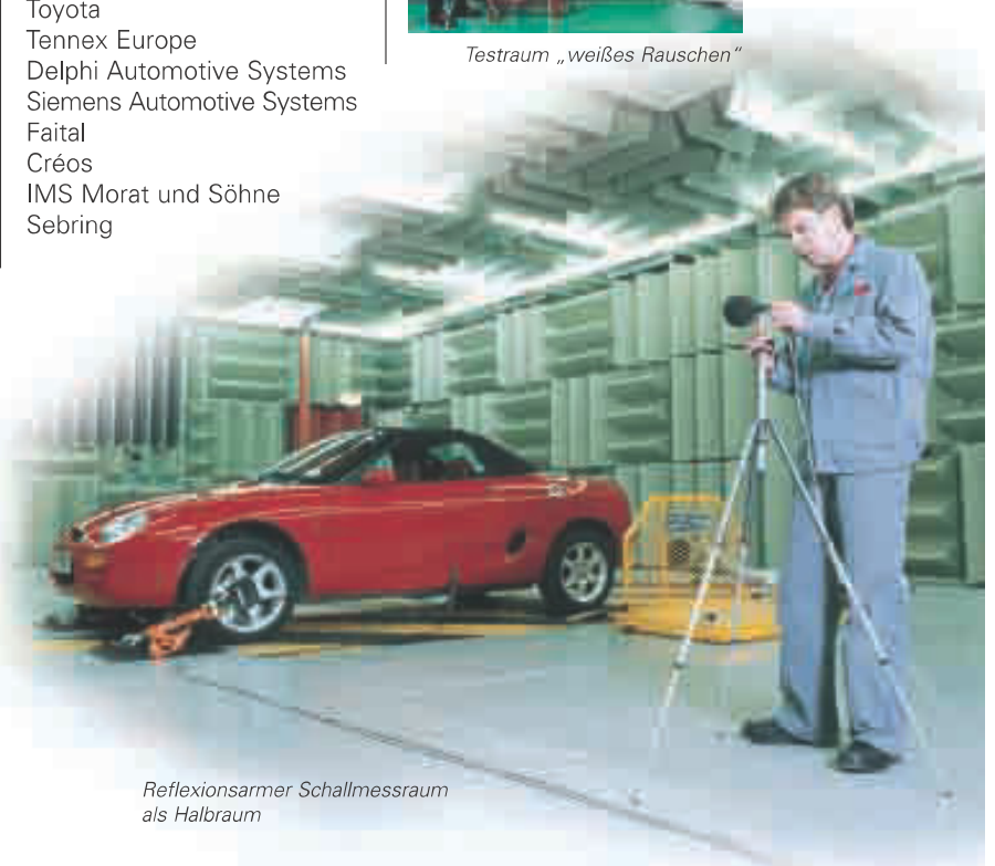
Reflexionsarmer Schallmessraum als Halbraum
